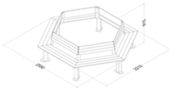
Banc ref 31460
