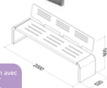
Banc ref 30171
