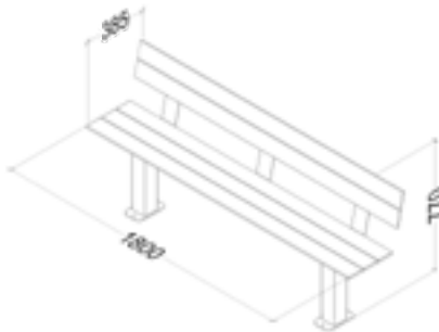
Banc ref 31221
