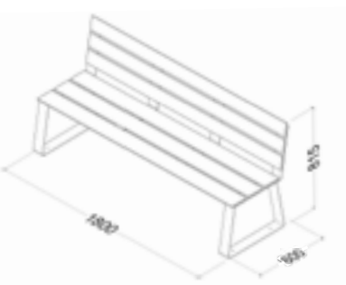
Banc ref 30571
